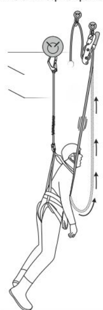
Рис. 4а. Предустановленная система, подъем
