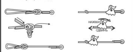
Рис. 7. Регулировка длины
