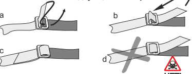
Рис. 4. Использование пряжек DUPLEX
