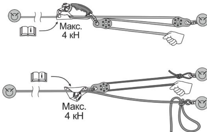
Рис. 4. Наведение переправы
